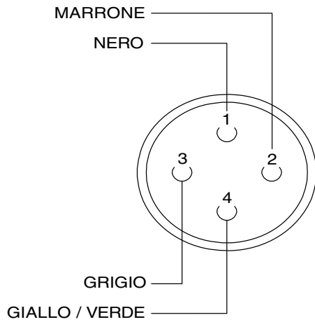
CONNETTORE ALIMENTAZIONE TRIFASE THREE-PHASE SUPPLY CONNECTOR
